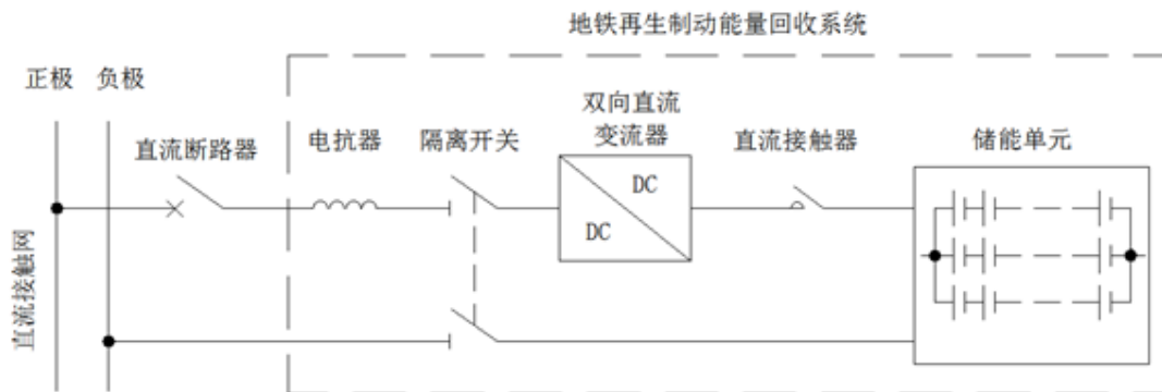
图 2 地铁再生制动能量回收系统电气系统回路图
