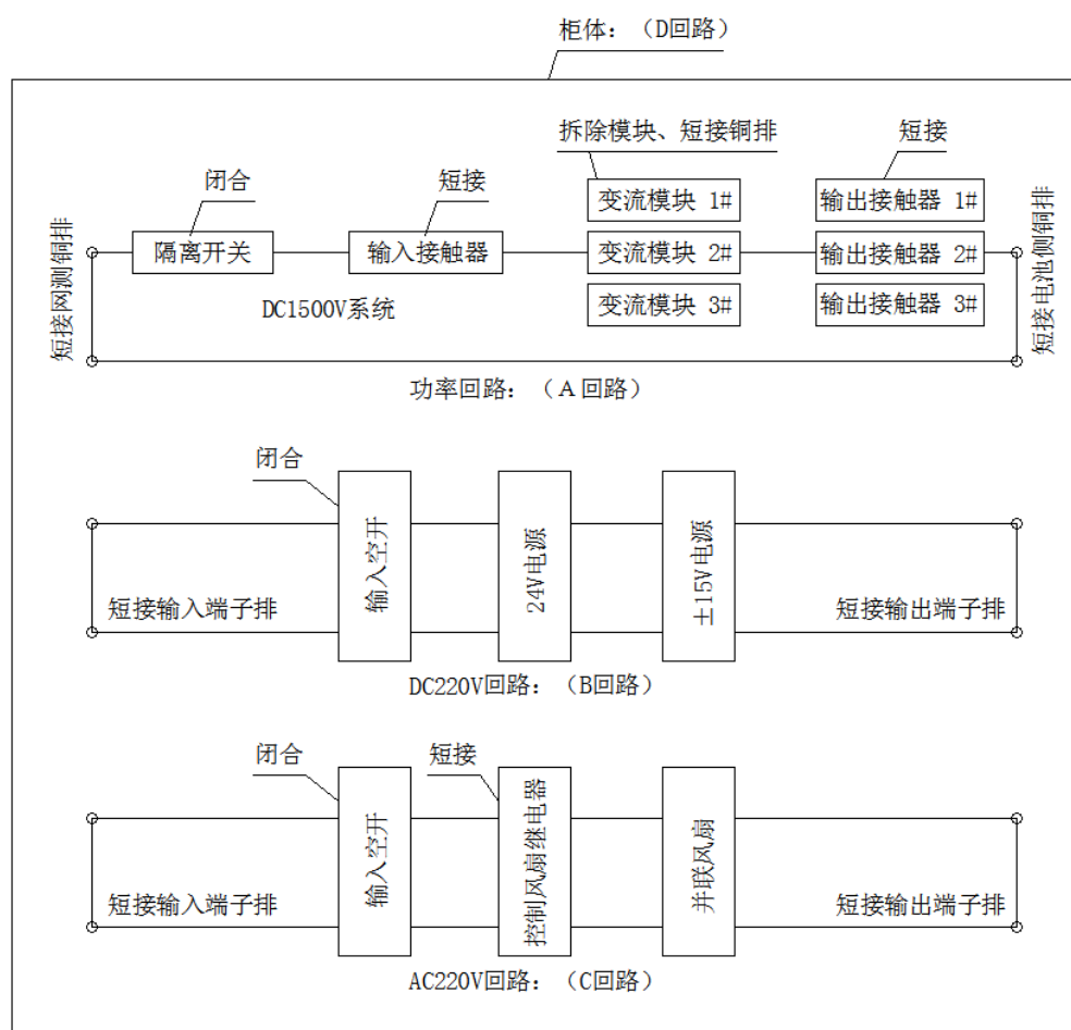
图4 绝缘试验电气联接图示
